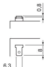
Type 2 Faston 6,3
