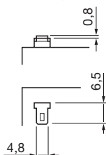
Type 1 Faston 4,8
